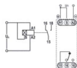
Ciclo iniziante con PAUSE Cycle beginning with PAUSE
