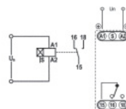
Ciclo iniziante con PULSE Cycle beginning with PULSE
